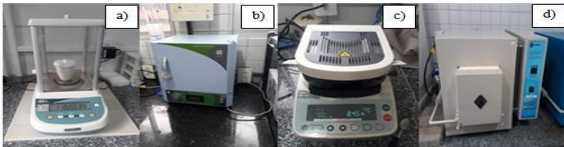
a) Balança de precisão; b) Estufa; c) Balança de umidade; d) Forno tipo mufla. Fonte: autores, 2019.
