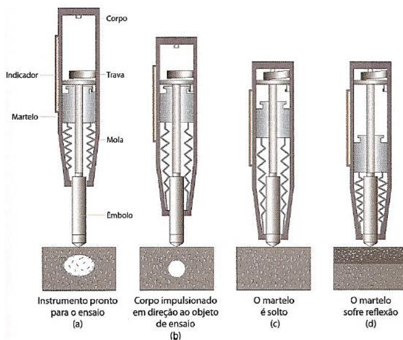
Figura 4: Esclerômetro - Esquema
