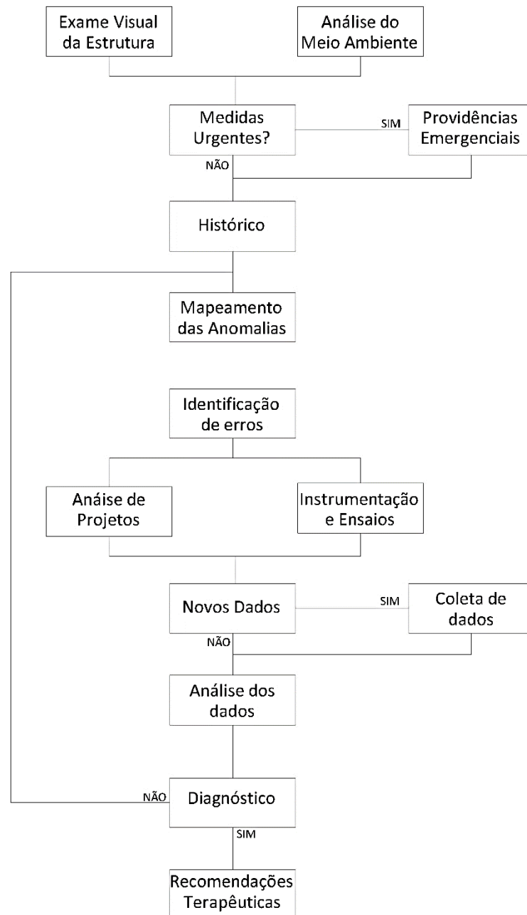
Figura 2: Fluxograma – Inspeção Visual de Estruturas
