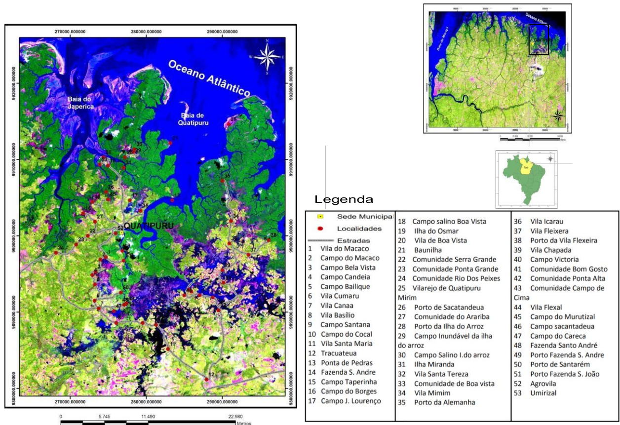
Figura 2 – Integração dos dados Vetoriais e Raster – Geoprocessamento do Geosistema de Quatipuru-PA
