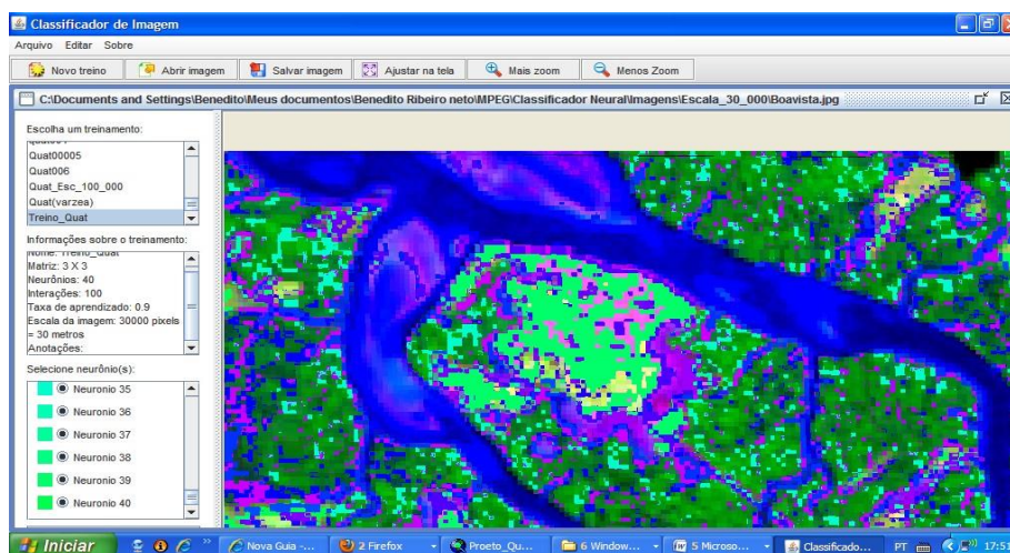
Figura 3 - Classificação das Unidades de Paisagem através do Classificador de imagens baseado em rede Neural artificial do LabGeo/IEC
