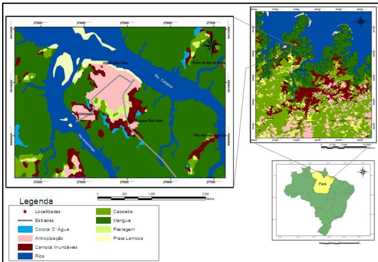
Figura 5 - Mapa da proporção Estuarina Mediana, caracterizado pela ocorrências das unidades de paisagens: manguezal, campo inundável, pastagem, antropização, capoeira, praia lamosa, rios e corpos D'água.
