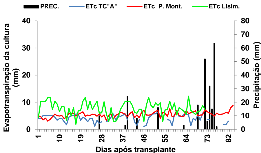
FIGURA 2. Precipitação e variação da evapotranspiração da cultura (mm) pelos métodos: Tanque Classe “A”, Penman-Monteith e medido por lisímetro durante o ciclo da cultura.
